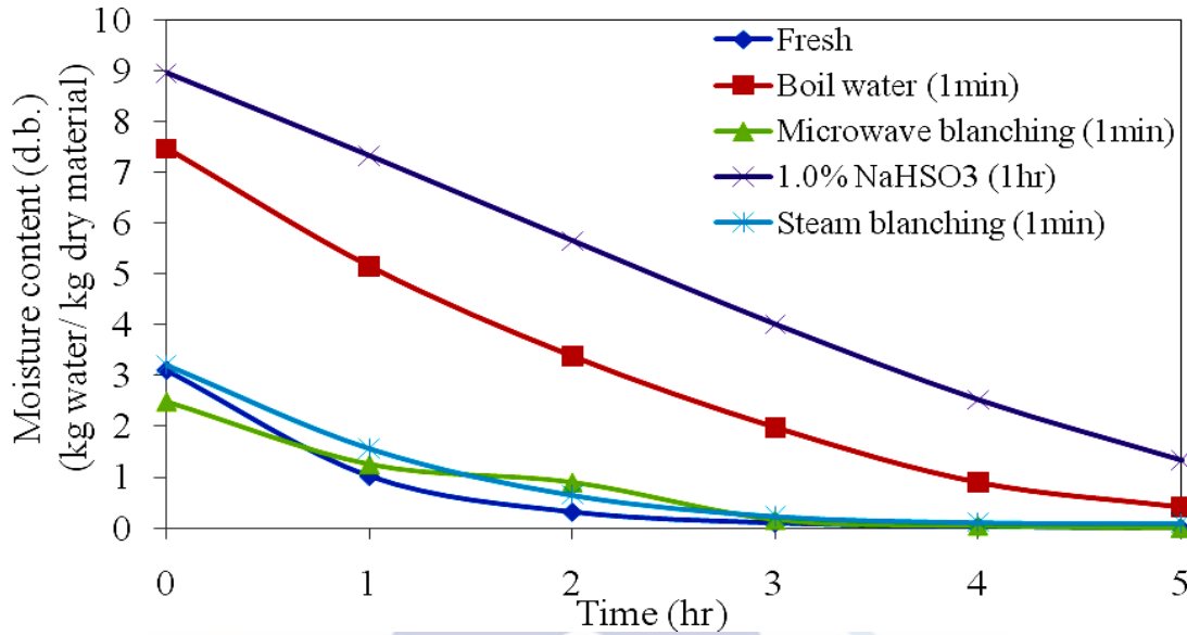
圖 1 不同前處理之雪耳熱風乾燥曲線(以乾基水分含量(d.b)表示)。
